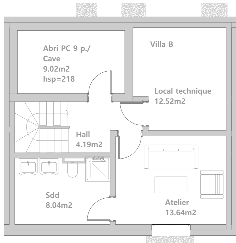
Villa B Sous-sol
