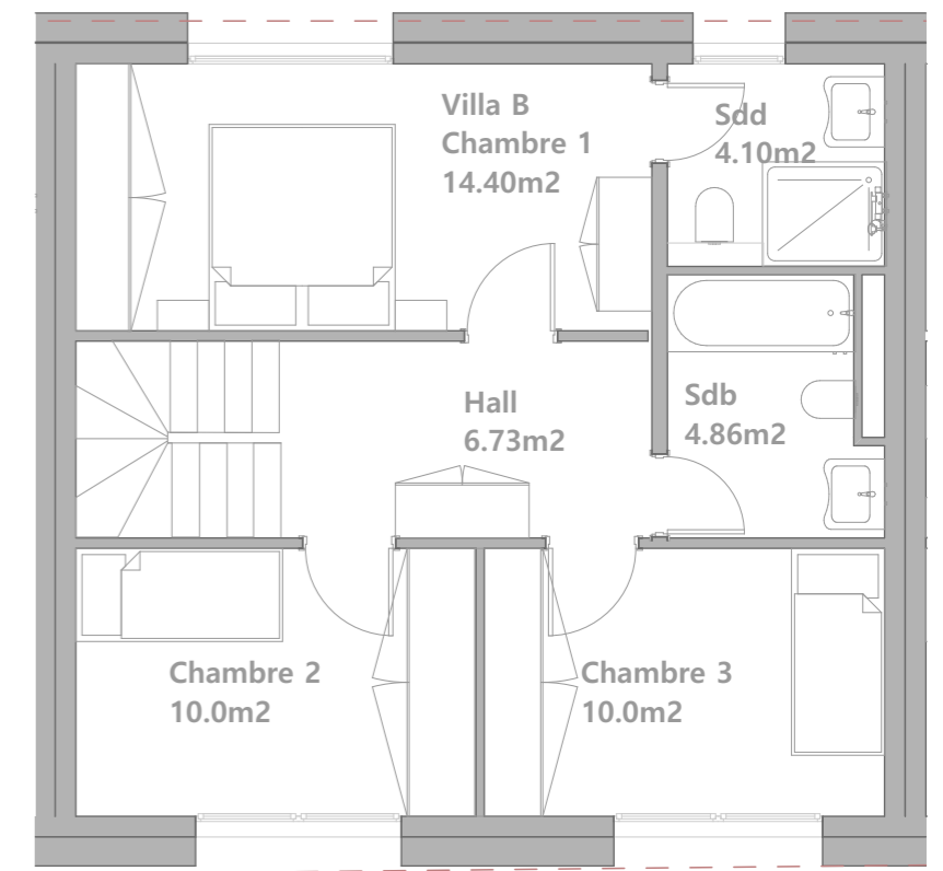
Villa B Etage 1
