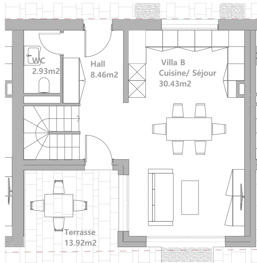
Villa B Rez de chaussee
